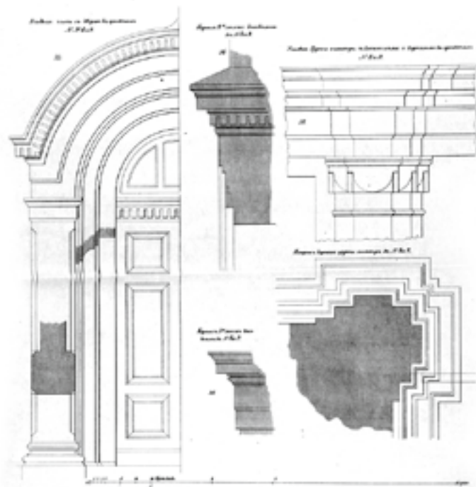
Детальные чертежи к проектам каменных церквей №№ 8 и 9. Составлены архитектором И.И. Свиязевым в 1861 г. РГИА.
