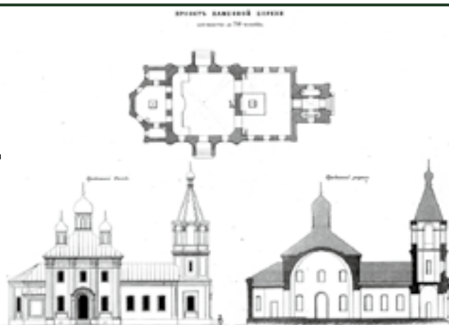
Проект каменной церкви вместимостью до 700 человек. № 9-й. [План.] Продольный фасад. Продольный разрез. Составлен архитектором И.И. Свиязевым в 1858 г. РГИА.
